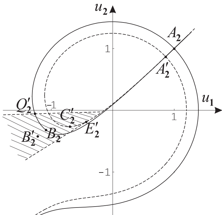
Рис. 2.9. Пример 3 ( \kappa > 0 )
