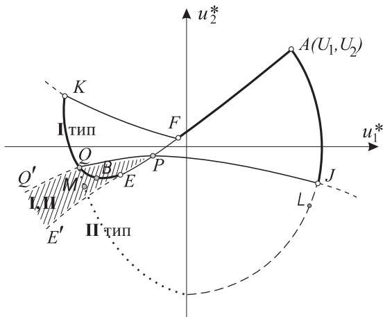
Рис. 1.4. Решение задачи о поршне для \kappa > 0 : зависимость решения от граничных данных u_\alpha|_{x=0} = u_\alpha^* при u_\alpha|_{t=0} = U_\alpha . Заштрихована область двужначности решения
