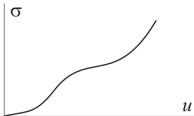
Рис. 4.1. \sigma(u)
