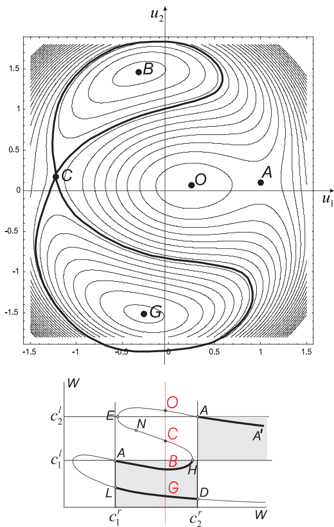
Рис. 3.6. Линии уровня ( \kappa < 0 )
