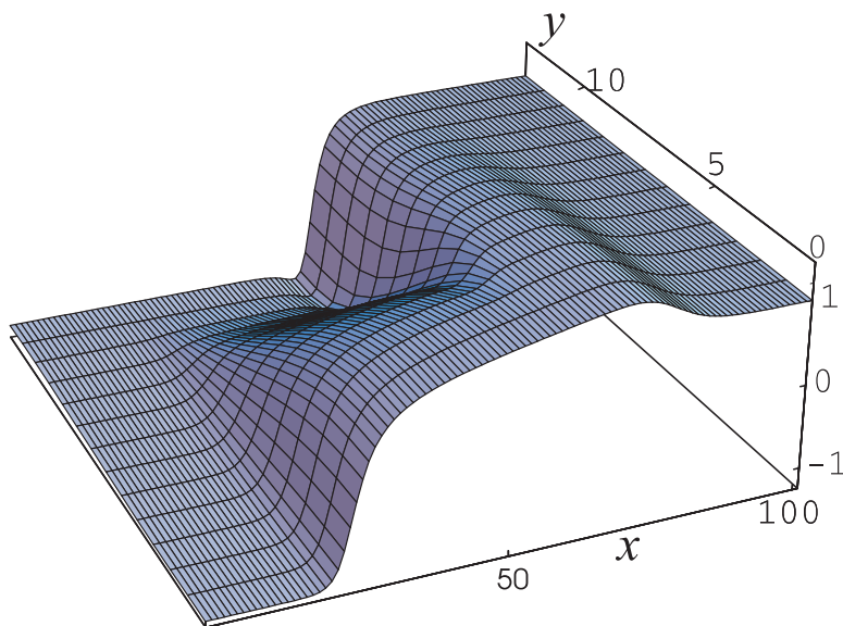
Рис. 2.18. Начальные данные, включающие “переходные зоны”
