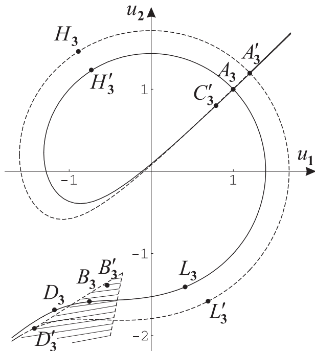
Рис. 2.10. Пример 4 ( \kappa < 0 )
