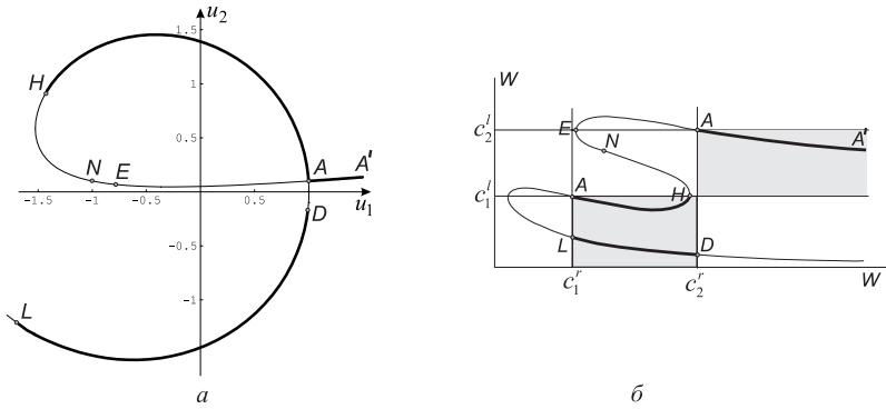
Рис. 1.3. Ударная адиабата и диаграмма эволюционности для для сред с \kappa < 0
