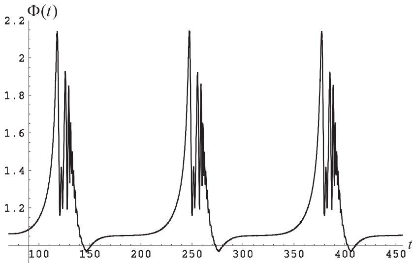
Рис. 4.6. \Phi(t) = \max_x u(x, t) – периодическая функция абсолютного максимума функции u(x, t)
