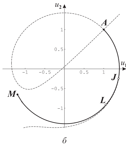
Рис. 2.4. Асимптотика автомодельного решения второго типа в средах с \kappa > 0
