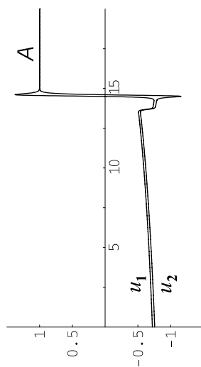
Рис. 2.14 в
