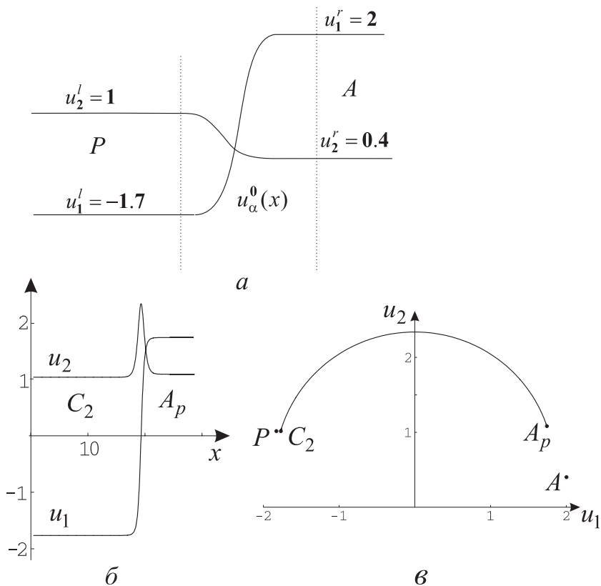
Рис. 3.12. Последовательность волн, представляющих решение примера 2 ( \kappa > 0 )
