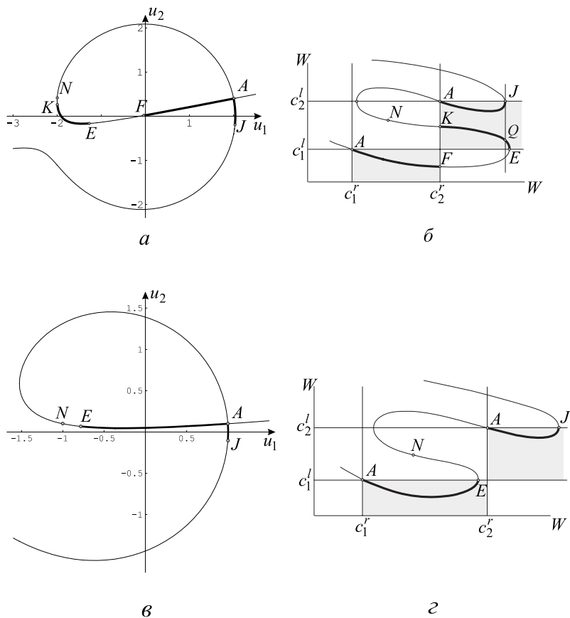
Рис. 1.2. Ударные адиабаты и диаграммы эволюционности для различных значений параметров g , \kappa , U_\alpha ( \kappa > 0 )
