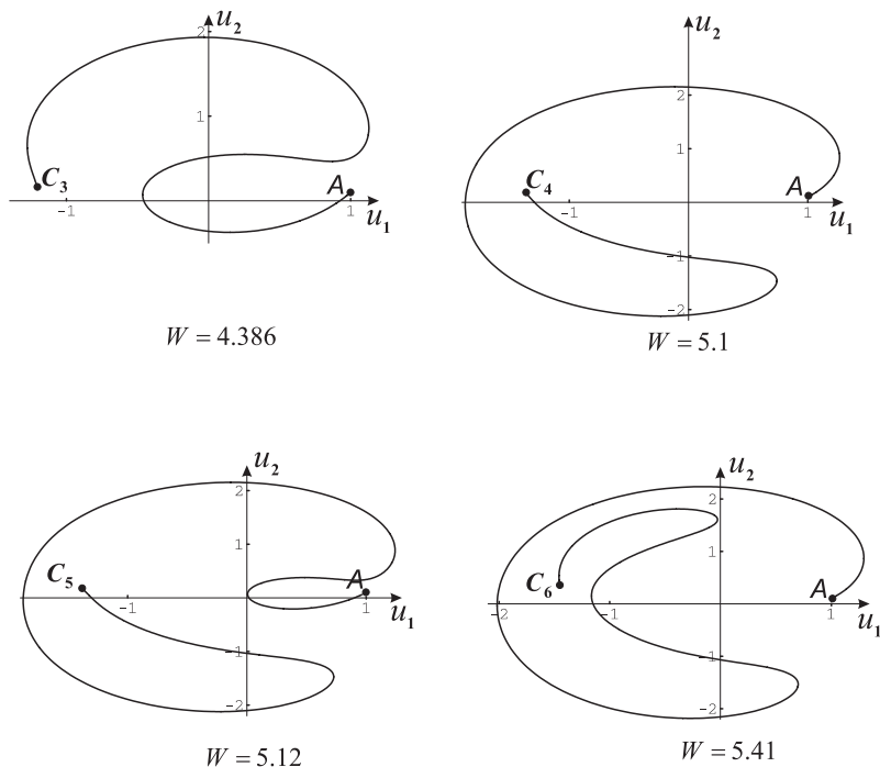
Рис. 3.9. Стационарные структуры особых разрывов ( \kappa < 0 )
