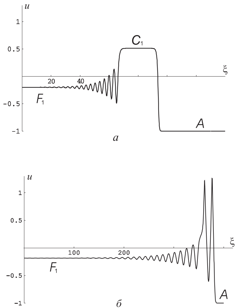
Рис. 4.4. Асимптотики решений уравнений в частных производных
