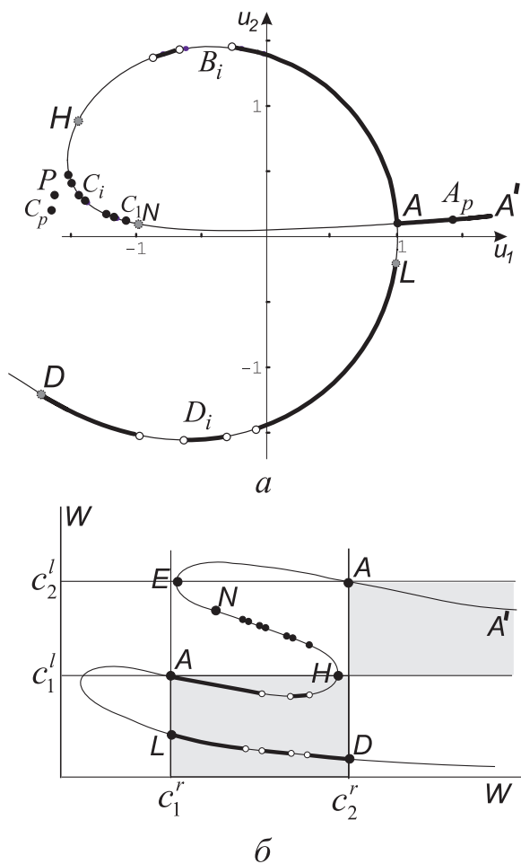
Рис. 3.10. Допустимая часть ударной адиабаты для волн в композитных материалах: жирные кривые и черные точки ( \kappa < 0 )
