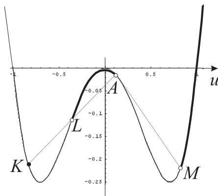
Рис. 4.2. \varphi(u) = u^4 - u^2
