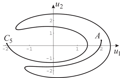
Рис. 3.4. Стационарные структуры особых разрывов ( \kappa > 0 )
