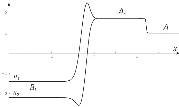
Рис. 2.5. Асимптотика автомодельного решения первого типа в средах с \kappa < 0
