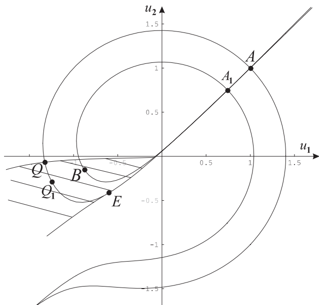
Рис. 2.6. Пример 1 ( \kappa > 0 )
