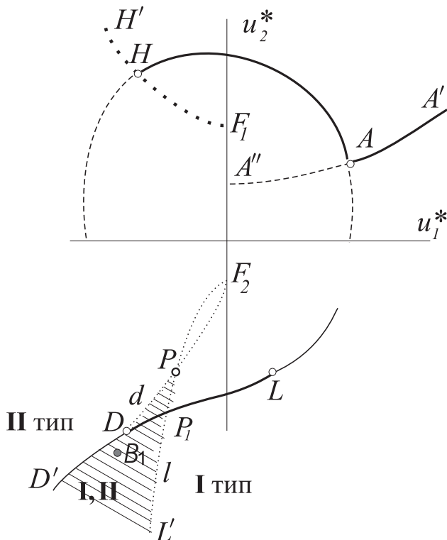
Рис. 1.5. Решение задачи о поршне для \kappa < 0 : зависимость решения от граничных данных u_\alpha|_{x=0} = u_\alpha^* при u_\alpha|_{t=0} = U_\alpha . Заштрихована область двужначности решения
