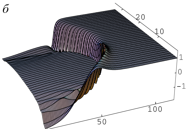
Рис. 2.20. Перестройка решения
