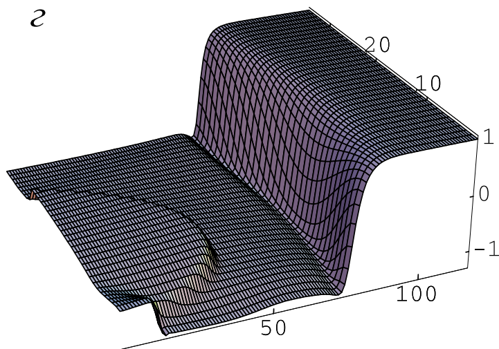
Рис. 2.20 (продолжение)
