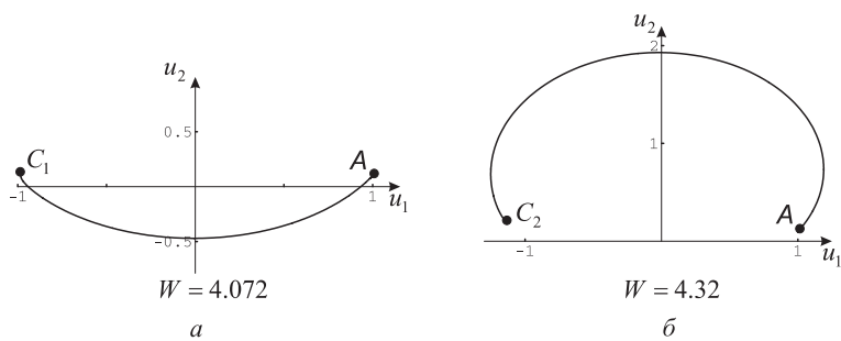
Рис. 3.8. Стационарные структуры особых разрывов ( \kappa < 0 )
