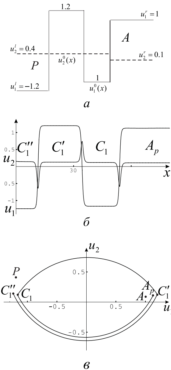
Рис. 3.17. Последовательность волн, представляющих решение при- мера 7 ( \kappa < 0 )
