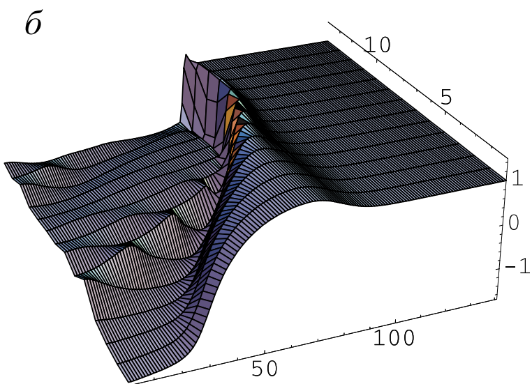
Рис. 2.19. Перестройка решения
