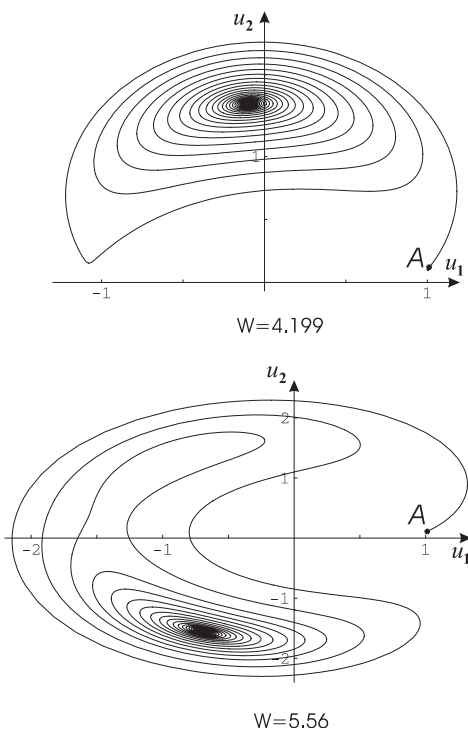
Рис. 3.7. Стационарные структуры разрывов ( \kappa < 0 )
