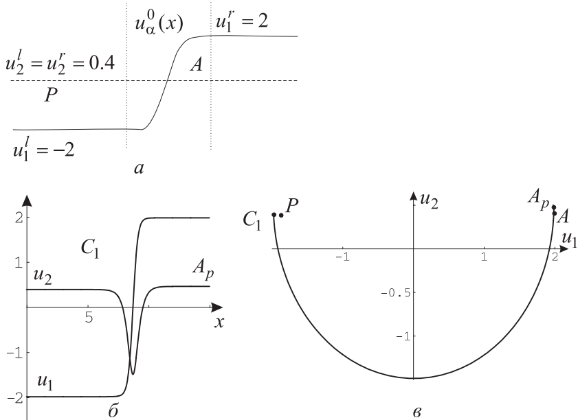
Рис. 3.11. Последовательность волн, представляющих решение примера 1 ( \kappa > 0 )
