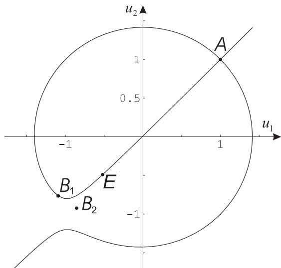
Рис. 2.12. Ударная адиабата для параметров \kappa = 1 , g = 0.01 , f = 1 , U_1 = U_2 = 1
