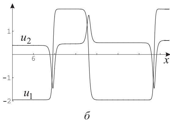
Рис. 3.13. Последовательность волн, представляющих решение при- мера 3 ( \kappa > 0 )
