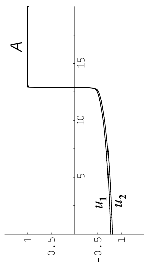
Рис. 2.14 б
