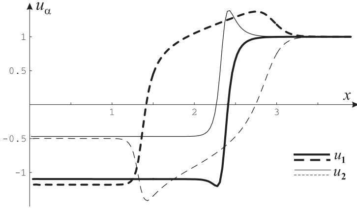
Рис. 2.17. Начальные данные
