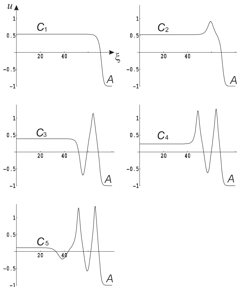
Рис. 4.3. Стационарные структуры
