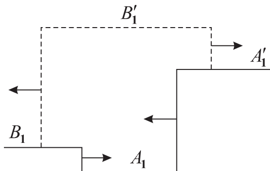
Рис. 2.7. Задача о взаимодействии двух ударных волн, движущихся навстречу друг другу
