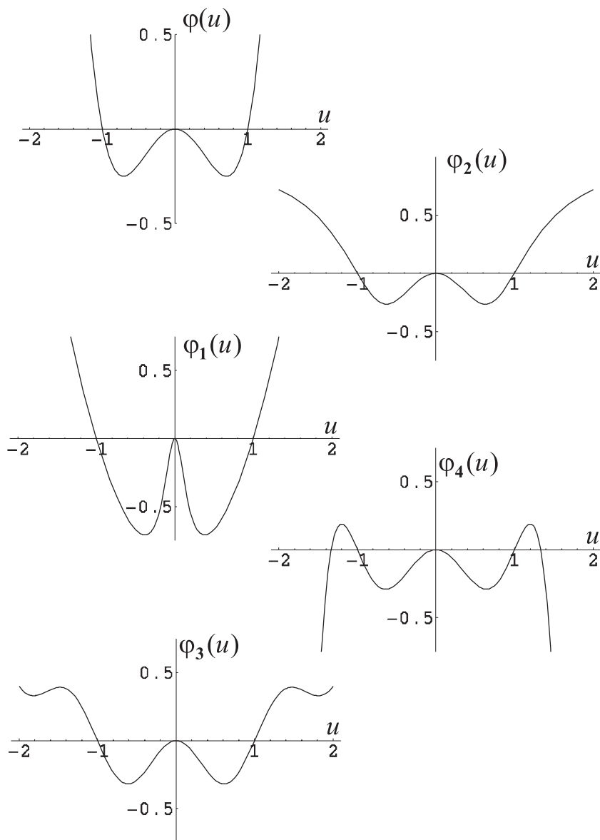
Рис. 4.7. \varphi_i(u)
