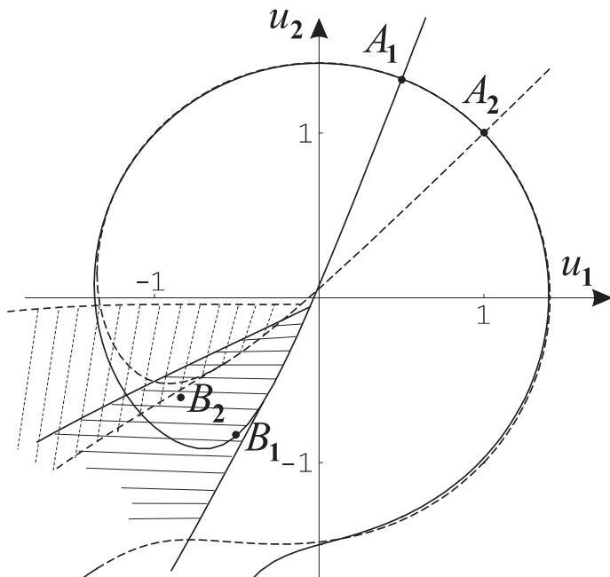
Рис. 2.16. Ударные адиабаты для начальных точек A_1(0.5, 1.33) (сплошная линия), A_2(1, 1) (штриховая линия)
