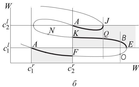
Рис. 2.1. Структура квазипоперечных ударных волн в средах с \kappa > 0
