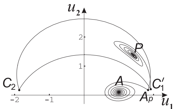
Рис. 3.16. Последовательность волн, представляющих решение при- мера 6 ( \kappa < 0 )
