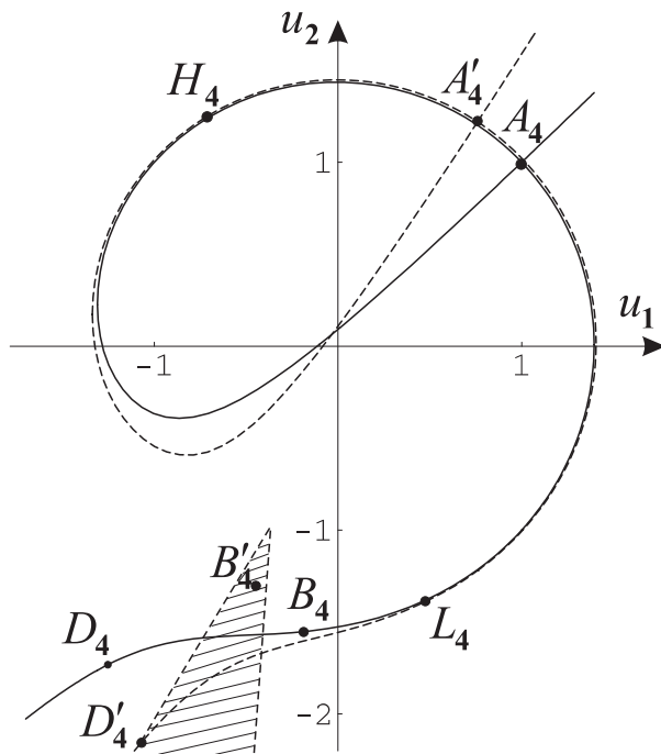
Рис. 2.11. Пример 5 ( \kappa < 0 )
