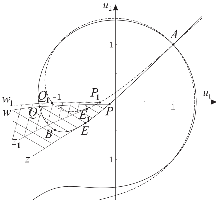
Рис. 2.15. Ударные адиабаты для параметров g = 0.03 (сплошная линия), g = 0.1 (штриховая линия)
