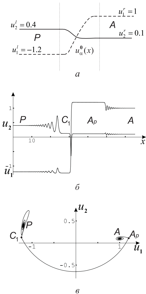
Рис. 3.14. Последовательность волн, представляющих решение при- мера 4 ( \kappa < 0 )
