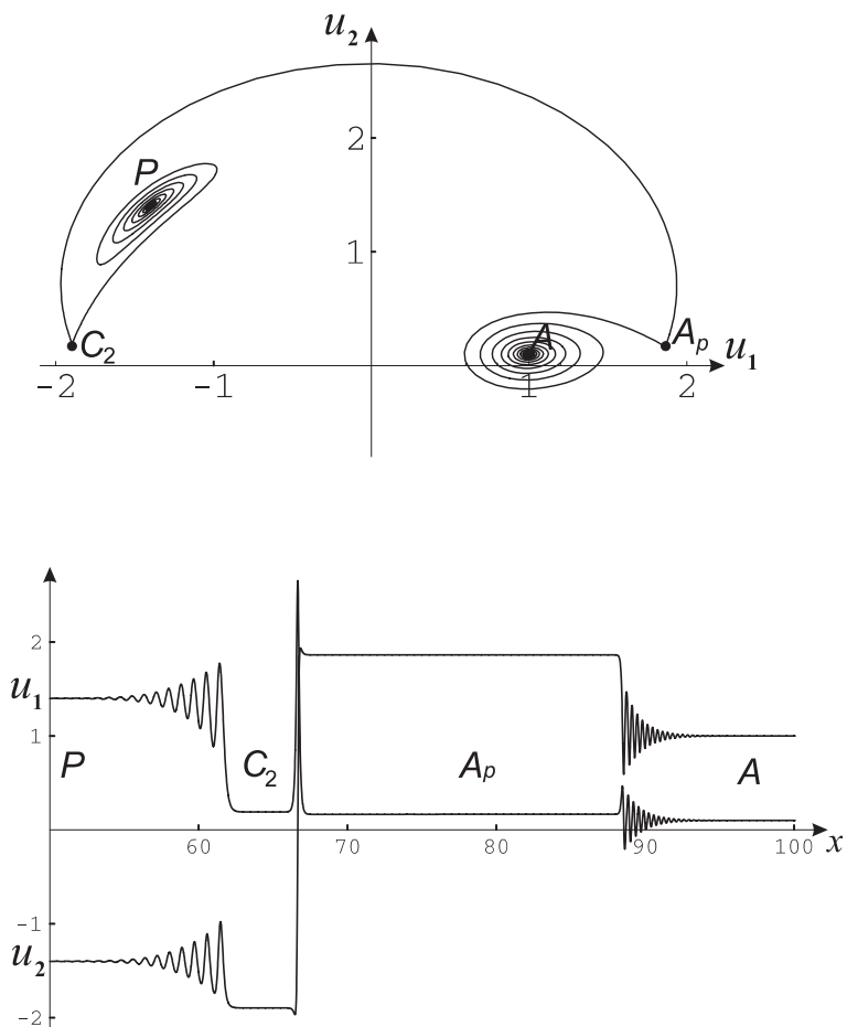
Рис. 3.15. Последовательность волн, представляющих решение примера 5 ( \kappa < 0 )
